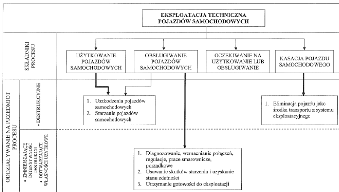
Rys. 2. Schemat procesu eksploatacji pojazdów samochodowych
