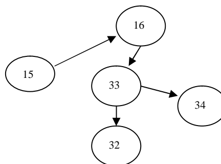
Рис.2. Орієнтовний граф, що показує логічні взаємозв'язки між поняттями сполук Карбону з теми „Неметалічні елементи та їхні сполуки”
