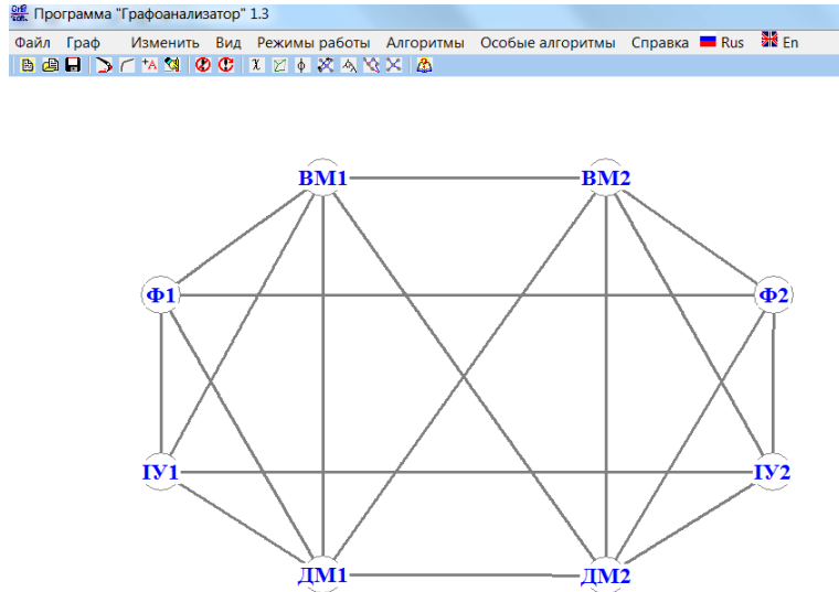
Рис. 1. Граф з заданими вершинами та ребрами
