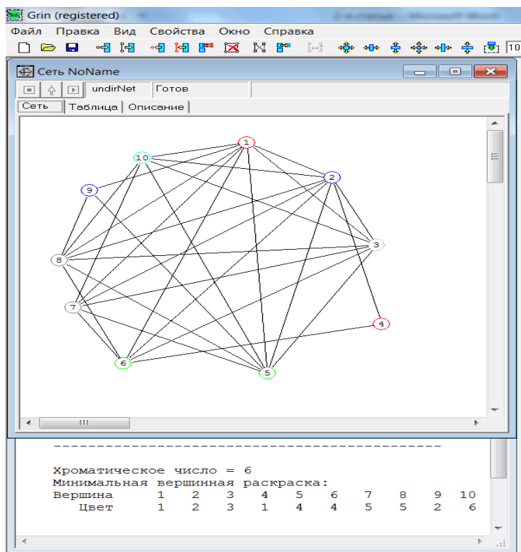
Рис. 5. Варіант розфарбування графа
