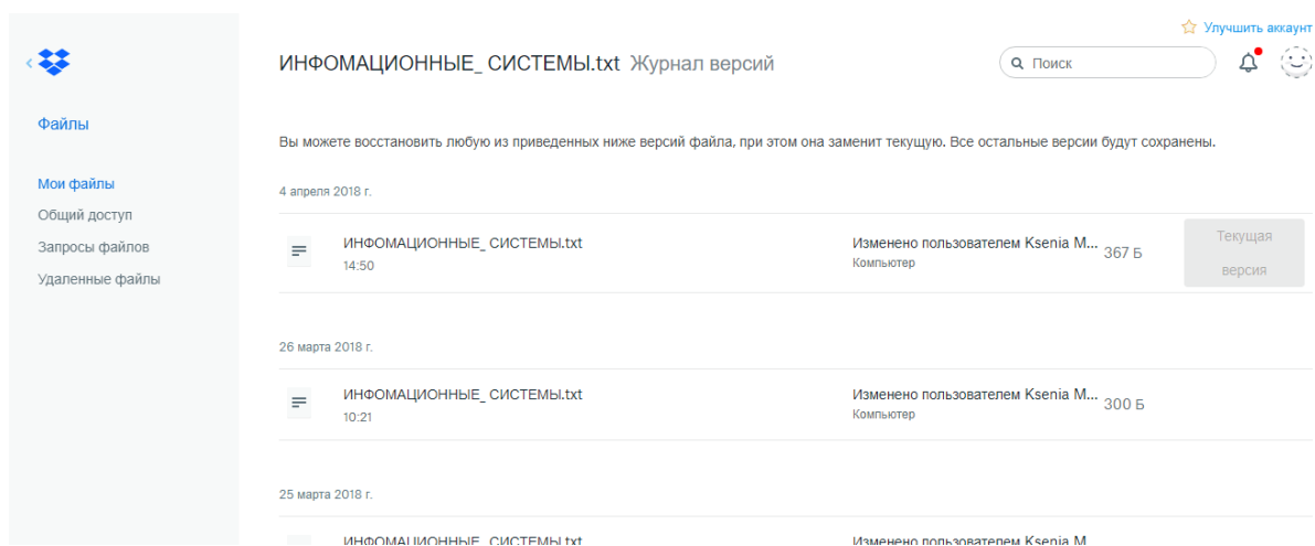
Рис. 2 – Журнал версий
