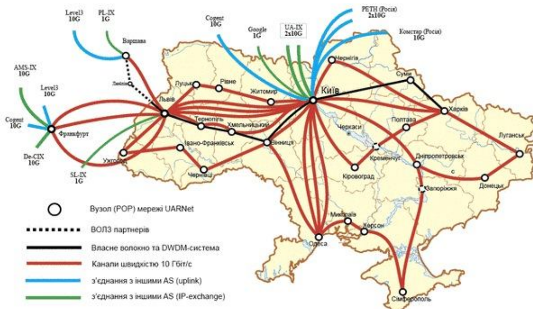
Рисунок 3. Топологія мережі UARNet станом на 2011 рік.
